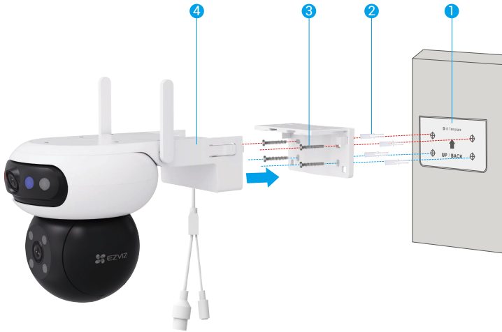
그림 2 벽 장착
